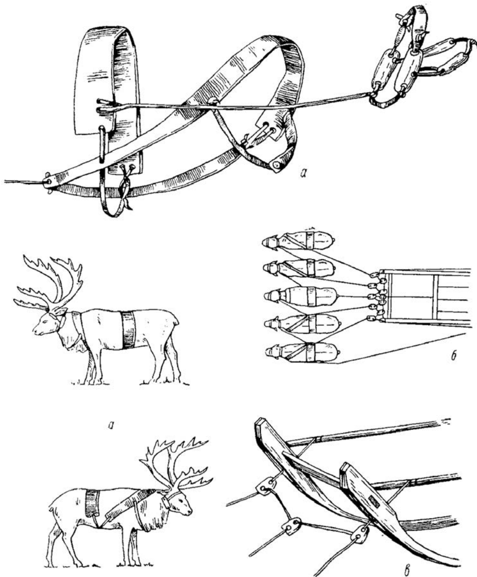
Рис. 27. Упряжь для легкой нарты: а) упряжь на одного оленя (не передового), б) упряжь на пять оленей, в) способ крепления быков к нарте
