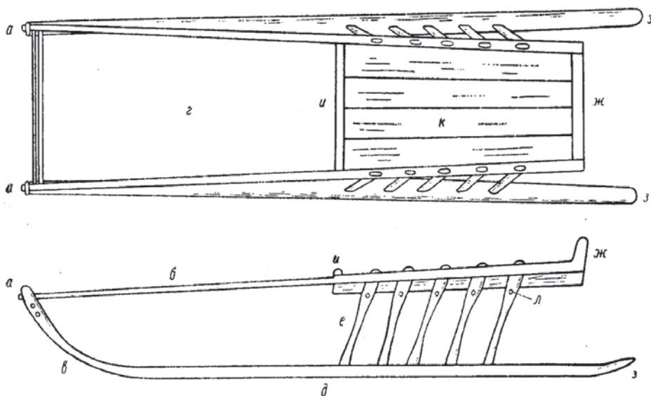
Рис. 25. Устройство нарты: а) хан' пья' (нос нарты), б) нин, в) харму', г) хан'лэхэ', д) ханз', е) хан' нгэ' (ноги нарты), ж) пуний тёндер', з) ябцо, и) нерний тёндер', к) хан' лата', л) нярт
