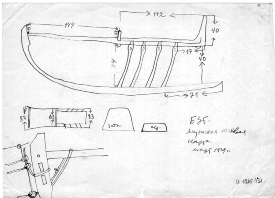
Рис. 15. Мужская легковая нарта. Большеземельская тундра. 1939. Рисунок Г.Д. Вербова. МАЭ И-1215-131
