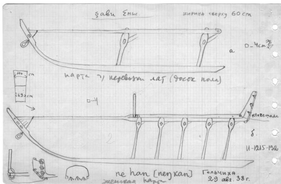
Рис. 17. şabu и neŋkan . Таймыр, р. Гольчиха. Рисунок Г.Д. Вербова. МАЭ И-1215-132
