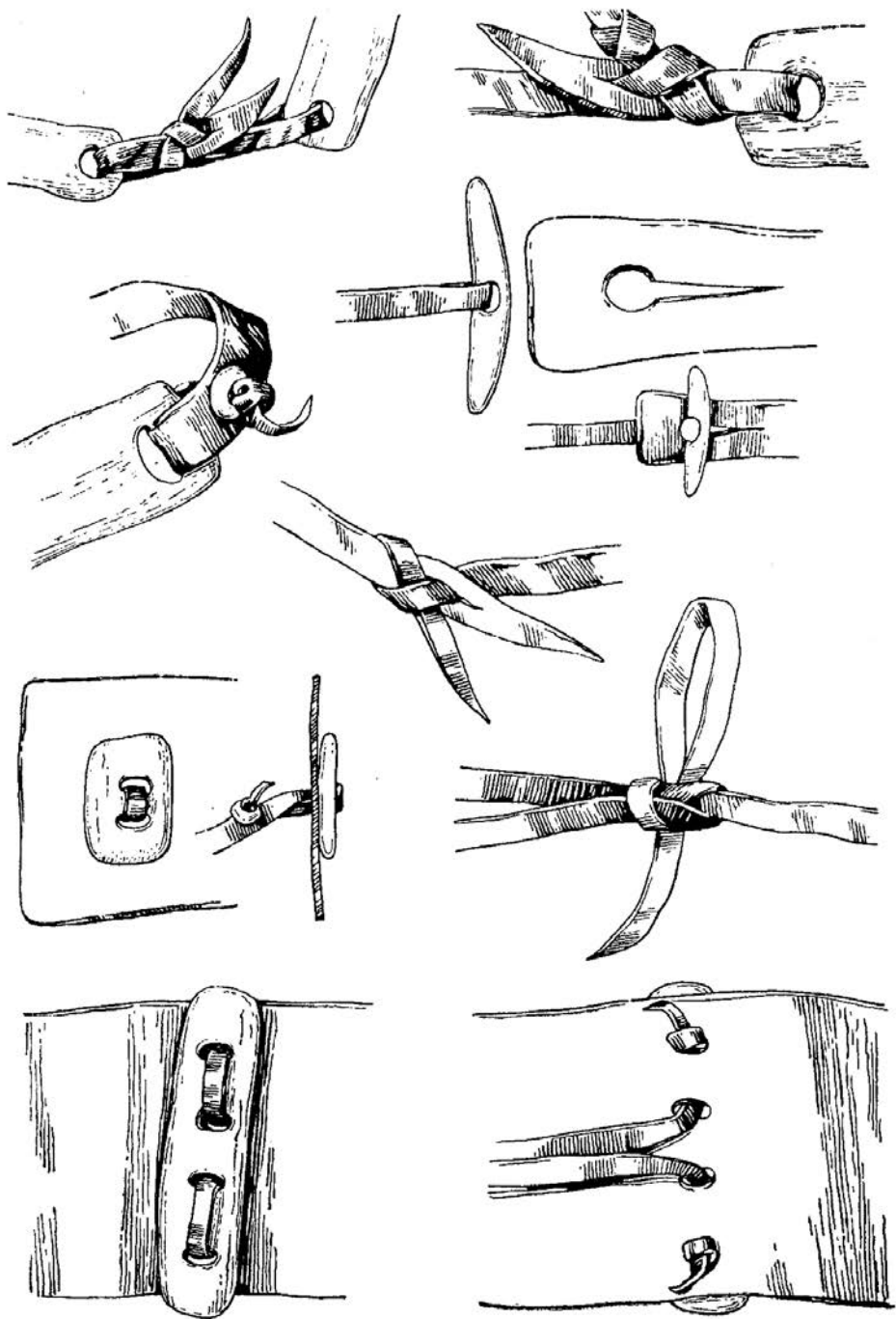
Рис. 29. Способы соединения частей упряжи
